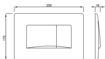
Tehnična risba
