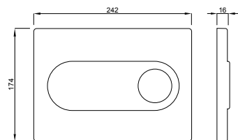
Tehnična risba
