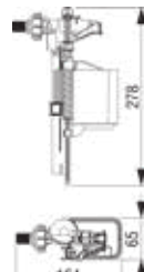
Tehnična risba
