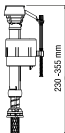
Tehnična risba
