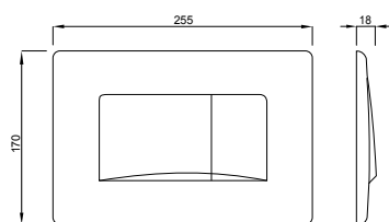
Tehnična risba
